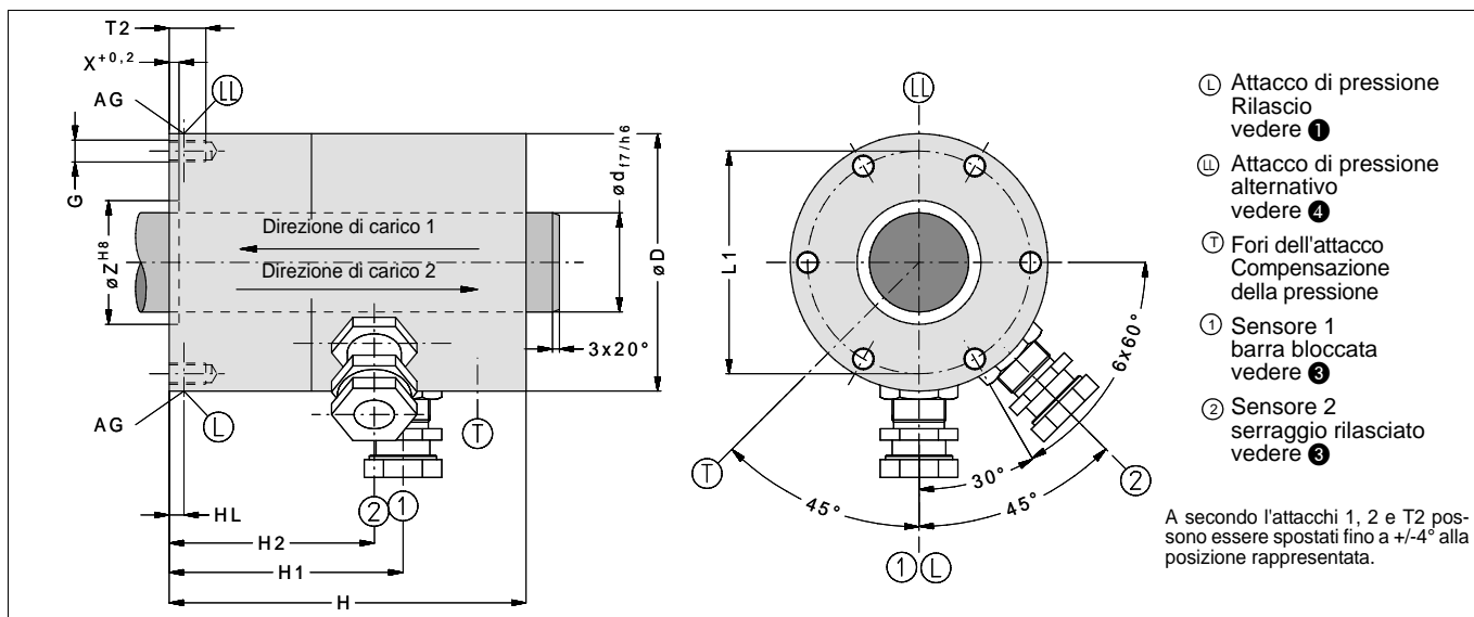
Fig. 1: Dimensioni dispositivo bidirezionale di arresto KFHW ( scaricare i file CAD dal sito Internet: www.sitema.com )
